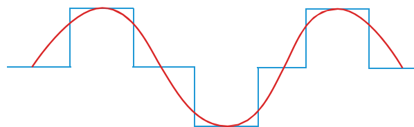
修正正弦波逆变器 纯正弦波逆变器
