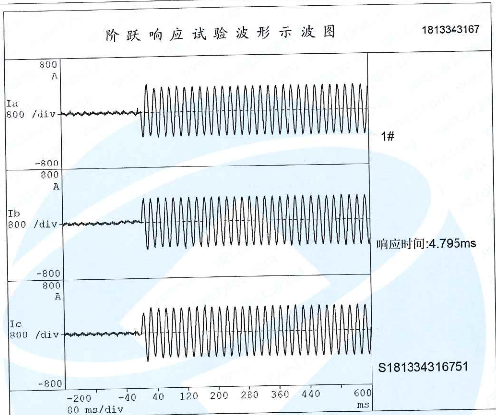
阶跃响应试验示波图
