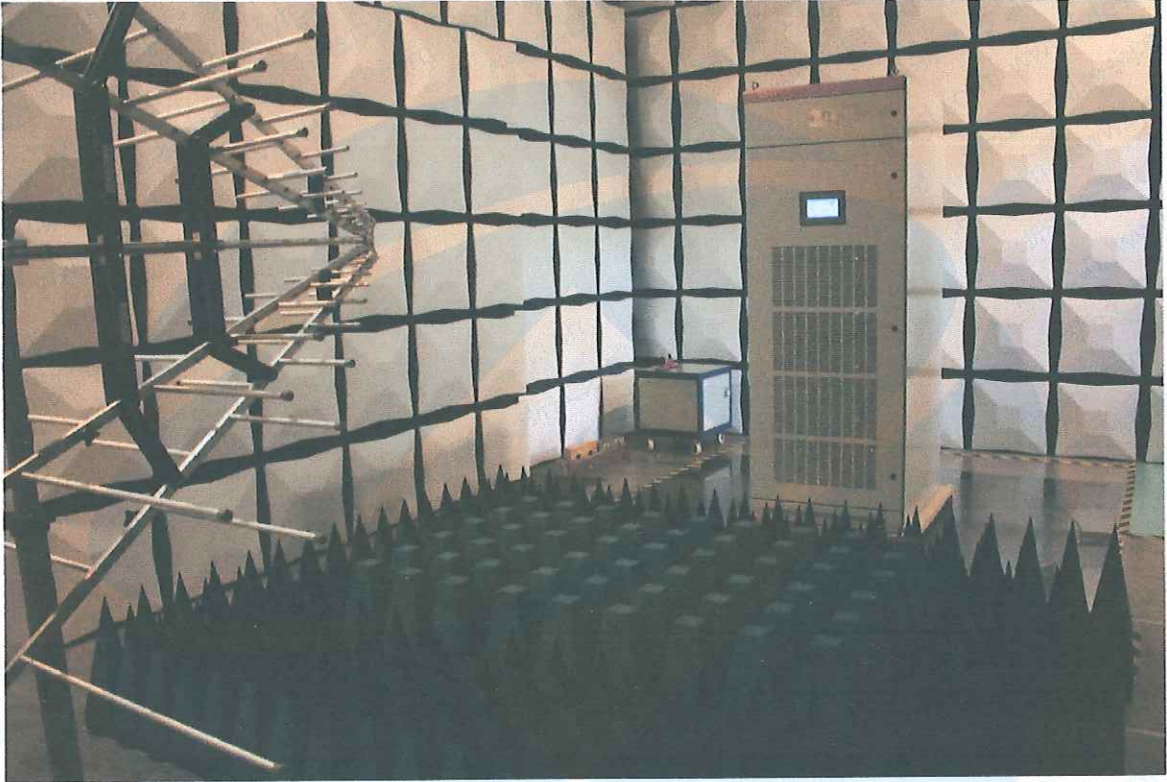
辐射电磁场干扰试验布置图:
