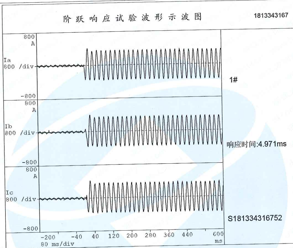
阶跃响应试验示波图
