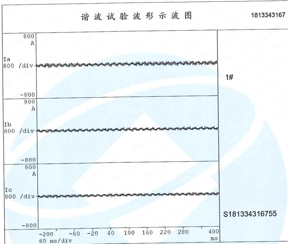
谐波试验示波图
