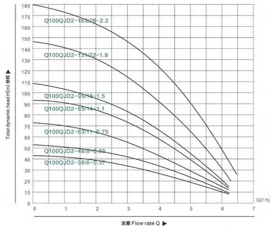
Q100QJ-2T性能参数表 PERFORMANCE TABLE
