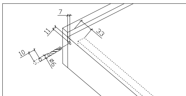
抽屉钻孔尺寸(mm)
