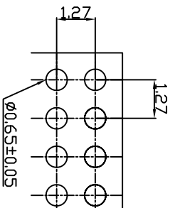
P.C.B Hole Layout
