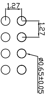
P.C.B Hole Layout
