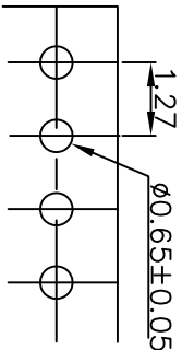
P.C.B Hole Layout
