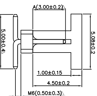
P.C.B. Hole Layout
