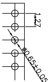
P.C.B Hole Layout
