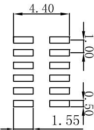
P. C. B SMT Layout
