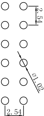
P.C.B.Layout
