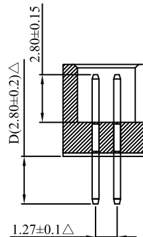
SEC:A-A
