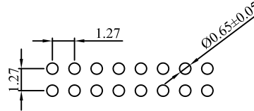
P.C.Board Layout
