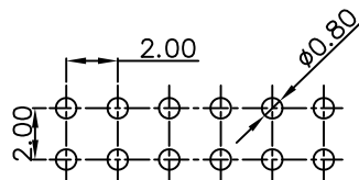
P.C.B Hole Layout
