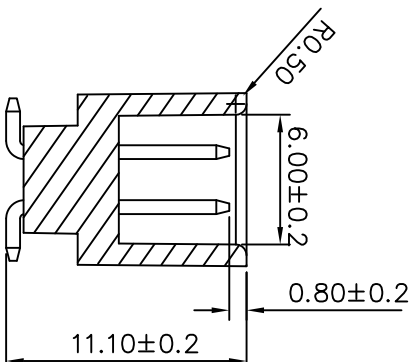
SEC A-A
