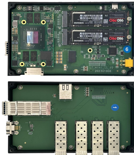
高速数据采集与储存FPGA直写NVMe SSD（双盘位） Высокоскоростной сбор и хранение данных: Прямая запись с FPGA на NVMe SSD (двухдисковый)
