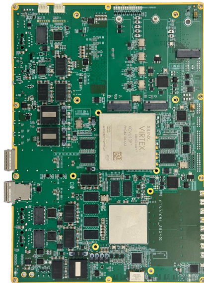
RTSD2501基带信号采 集处理板 Плата сбора и обработки СИГНАЛОВ ОСНОВНОЙ ПОЛОСЫ ЧАСТОТ RTSD2501
