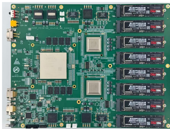
高速数据采集与储存FPGA直写NVMe SSD（八盘位） Высокоскоростной сбор и хранение данных: Прямая запись FPGA на NVMe SSD (8 дисков)
