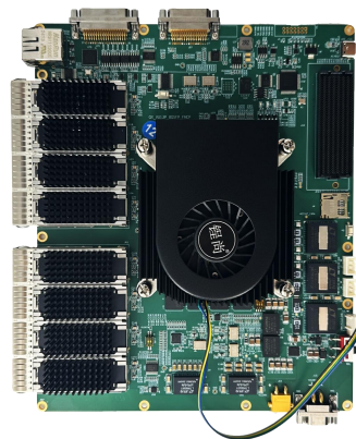
VU13P-FMC信号处理板 Плата обработки сигналов VU13P- FMC
