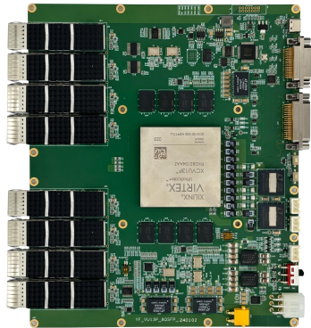
VU13P信号处理板 Плата обработки сигналов VU13P
