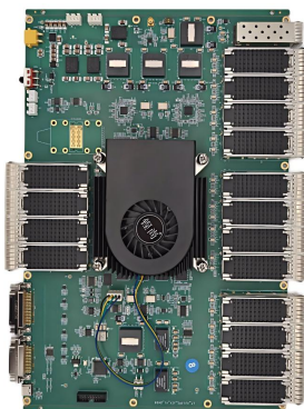
VU13P降采样信号处理板 Плата обработки сигнала с понижающей дискретизацией VU13P
