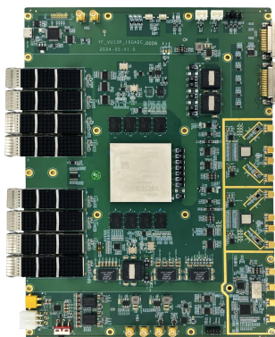
信号处理板 Двухканальная плата АЦП 10G + обработки сигнала
