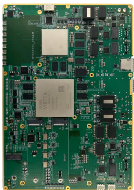
VU13P降采样信号处理板 Плата обработки сигнала с понижающей дискретизацией VU13P
